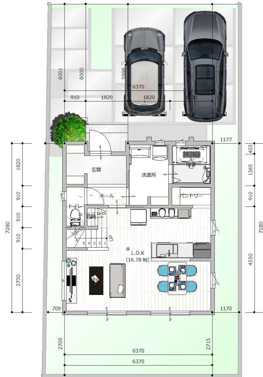
敷地図 1/100
