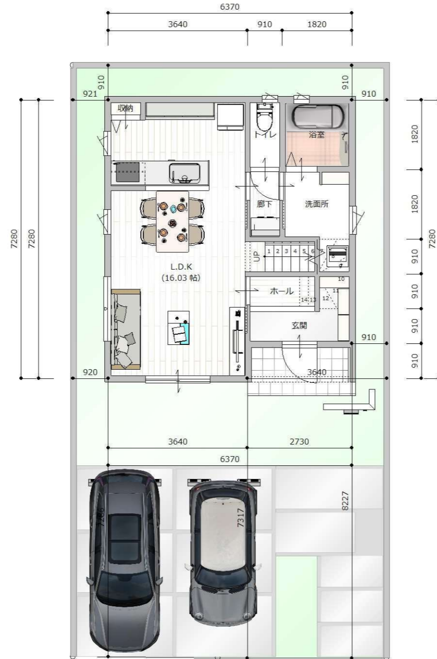
敷地図 1/100
