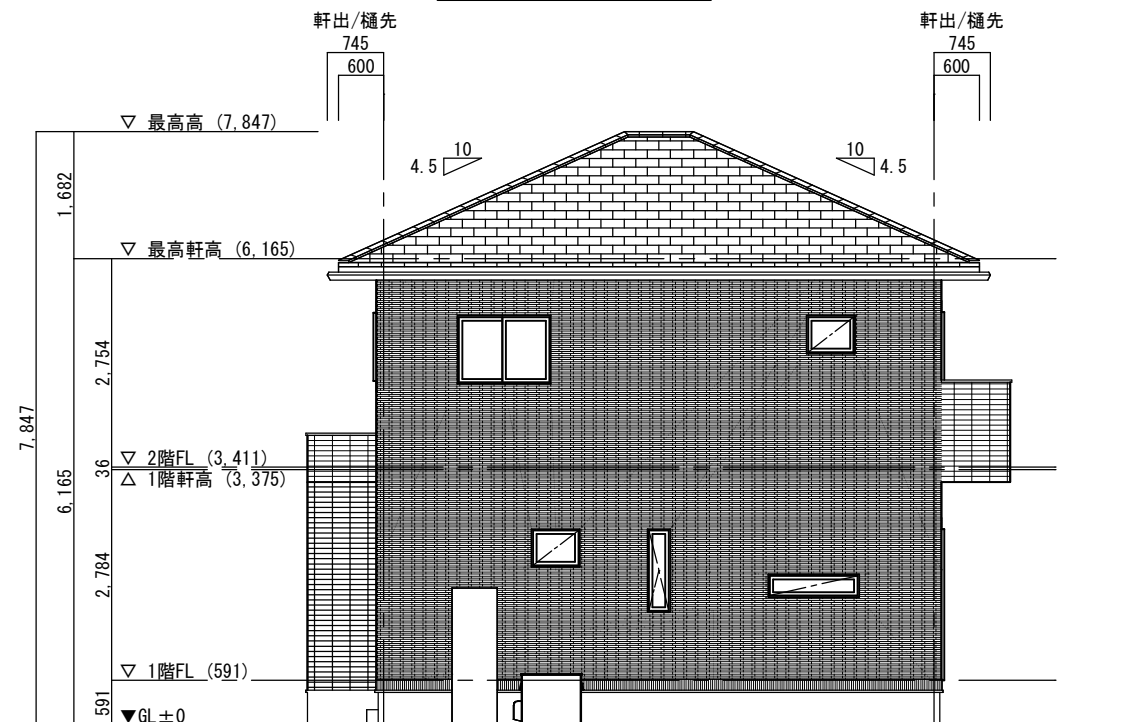
東側立面図
