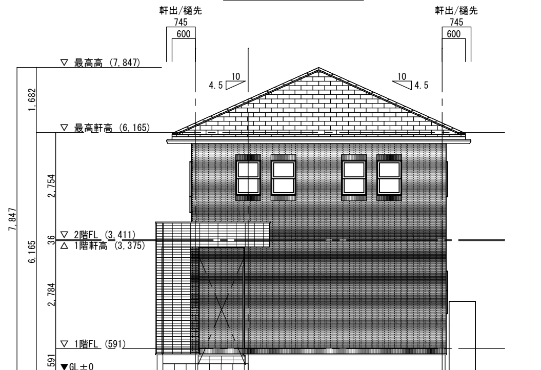
南側立面図
